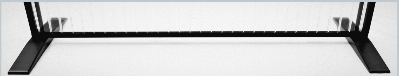
R2-Basis Set, Farbe anthrazit, 2 Standfüße R2-Basis, 2 U-Seitenprofile 2.000mm, 2 U-Stirnprofile mit Lochung 980mm oder 1.200mm (ohne Stegplatte)
